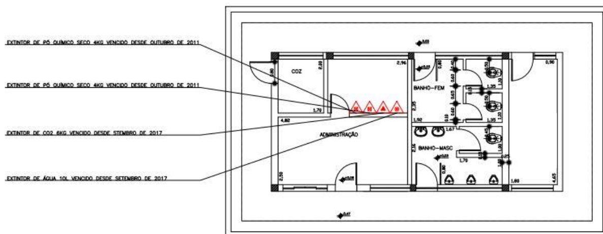
PLANTA esc. 1:50
